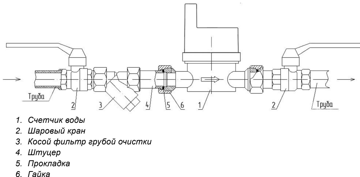
Рисунок 9 — Рекомендуемая схема монтажа
