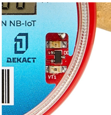
Рисунок 8 — Оптический порт
